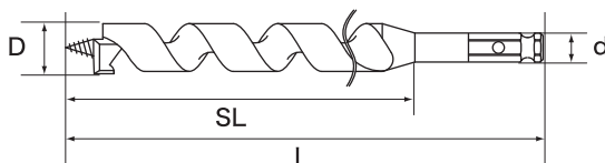
呼称サイズ:D 全長:L ネジ丈:SL 軸径:d (単位:mm)
