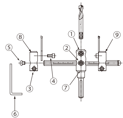
品番 36D ダイヤモンド自在錐
