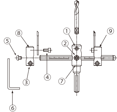
品番 36T 超硬自在錐
