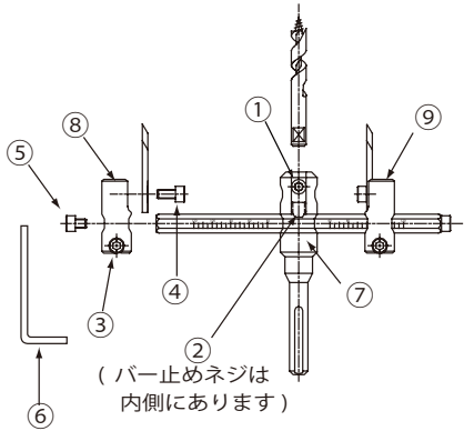
品番 36 自在錐
