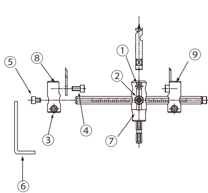
品番 36X 充電ドリル自在錐
