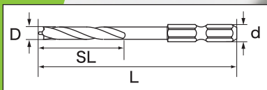
サイズ(mm):D 寸法(mm):全長Lxネジ丈SLx軸径d
