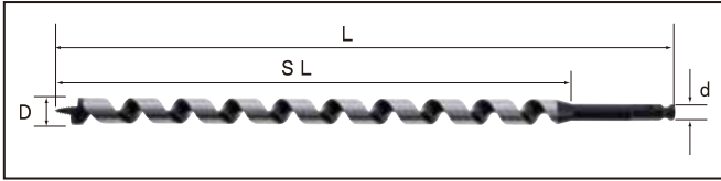
サイズ=D 全長=L ネジ丈=SL 軸径=d
