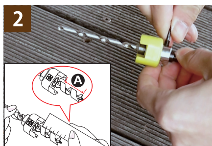
定規で穴あけ深さを決め、止めネジはボディではなく溝部分でしっかりと締め付ける
