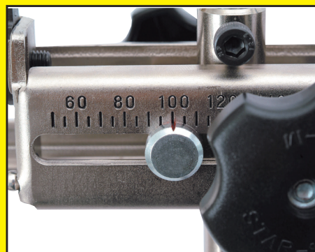
③穴径 100mm に合わせる場合、目盛りの赤線とフレームの数字を合わせ黒ハンドルをしっかり締め付ける。
