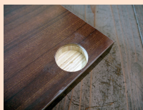
スライド丁番のカップ径に合わせて丁番錐で穴あけをする。
