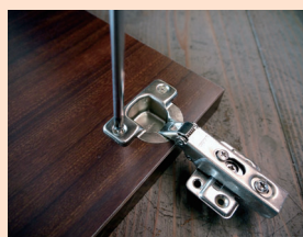
加工穴にスライド丁番をはめ込みネジを締め付ける。
