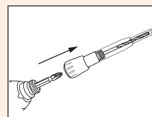
④本体を取り外す
